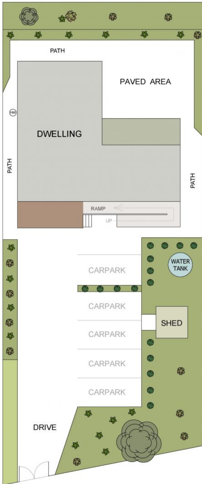
SITE PLAN (Land Size 841 sq m) Scale - 1:165
