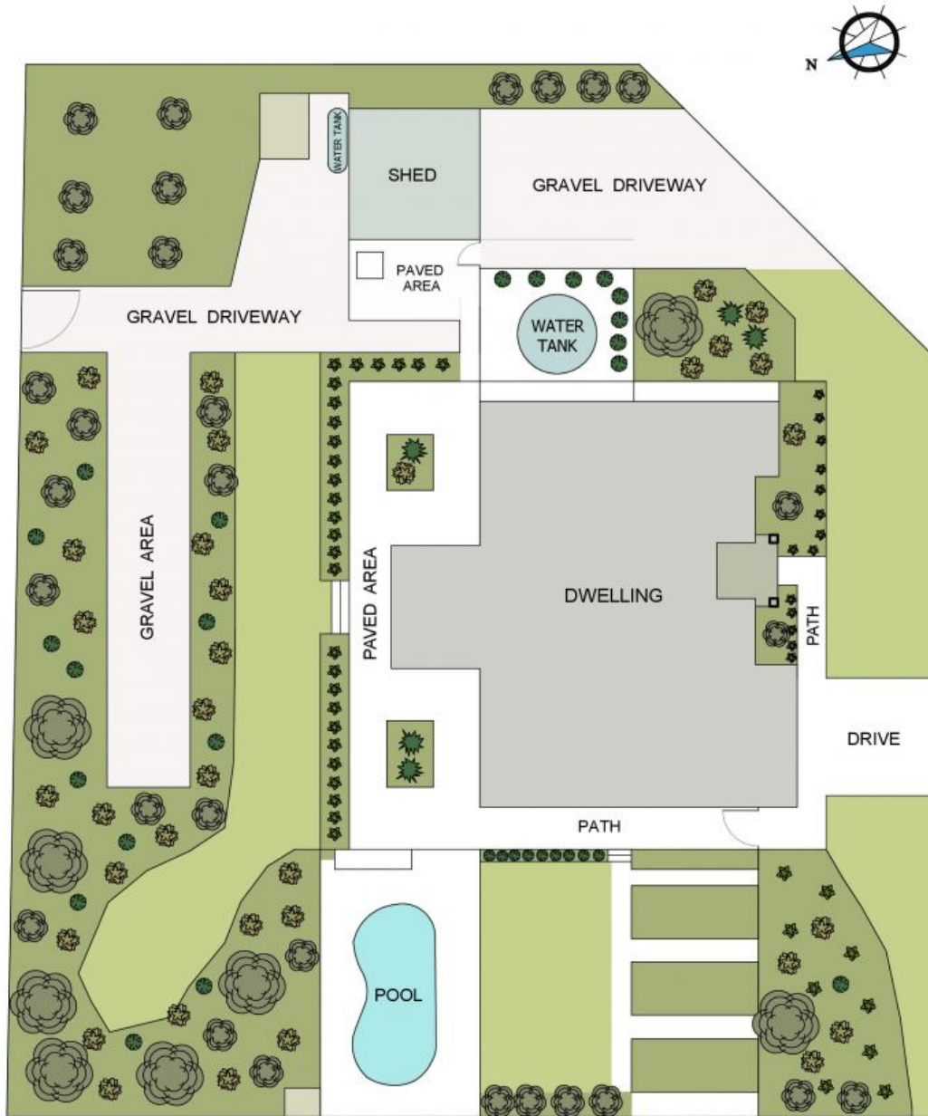
SITE PLAN (Land size - 2033 sq m) Scale - 1:335
